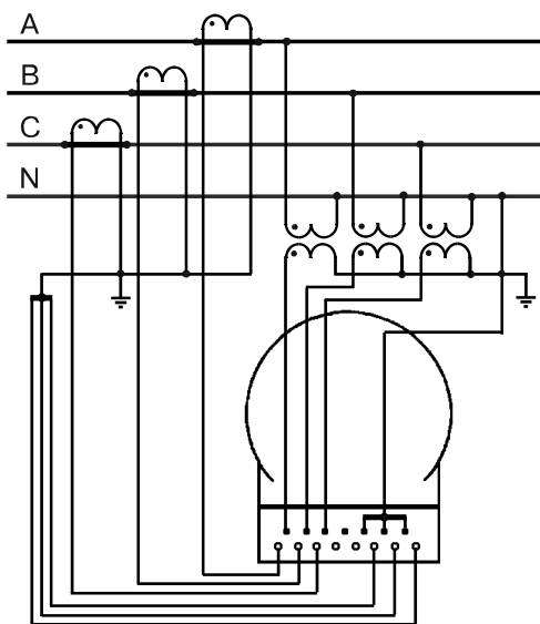
Рисунок 9 – Трехфазная четырехпроводная сеть с подключением через трансформаторы тока и напряжения
