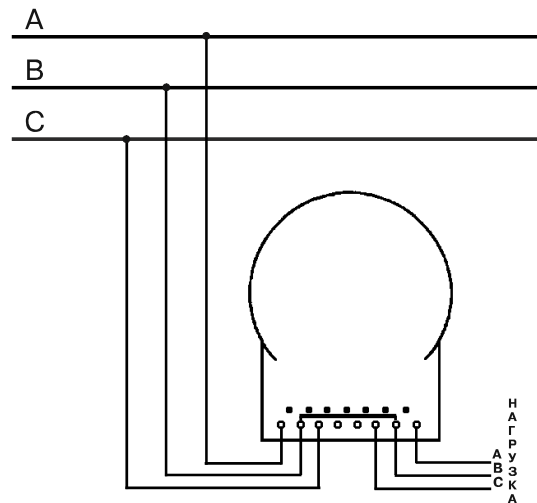
Рисунок 15 – Трехфазная трехпроводная сеть (двухэлементные счетчики)
