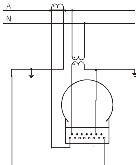
Рисунок 12 – Однофазная сеть с подключением через трансформаторы тока и напряжения
