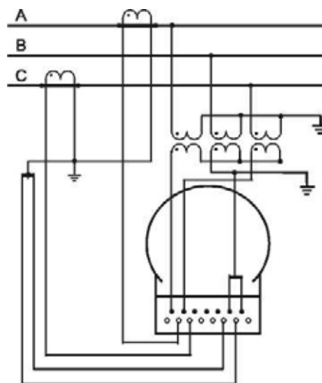
Рисунок 7 – Трехфазная трехпроводная сеть с подключением через трансформаторы тока и напряжения
