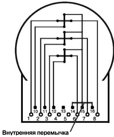
Рисунок 13 - Внутренние подсоединения токовых цепей и цепей напряжения к клеммнику счетчика
