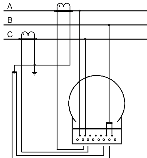
Рисунок 6 – Трехфазная трехпроводная сеть с подключением через трансформаторы тока
