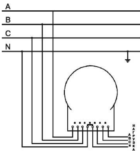
Рисунок 14 – Трехфазная четырехпроводная сеть (трехэлементные счетчики)
