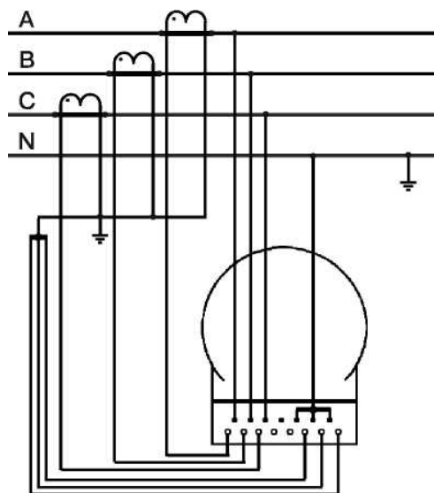
Рисунок 10 - Трехфазная четырехпроводная сеть с подключением через трансформаторы тока
