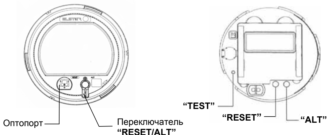
Рисунок 1 – Расположение кнопок и переключателя счетчика
