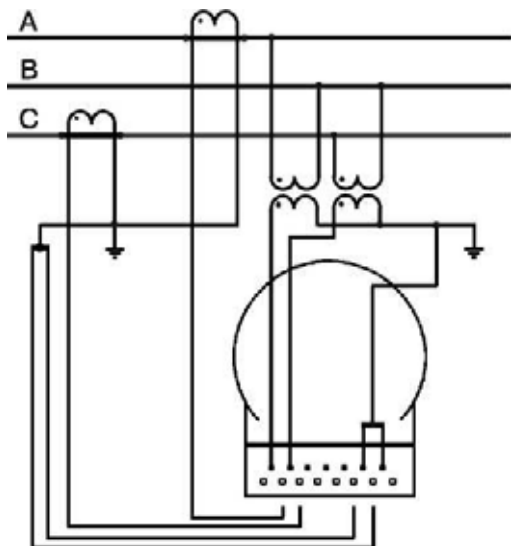
Рисунок 5 – Трехфазная трехпроводная сеть с подключением через трансформаторы тока и напряжения
