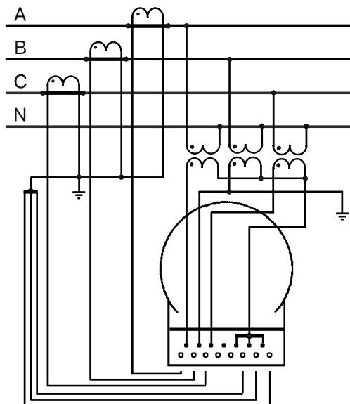
Рисунок 11 - Трехфазная четырехпроводная сеть с изолированной нейтралью и заземленной фазой В
